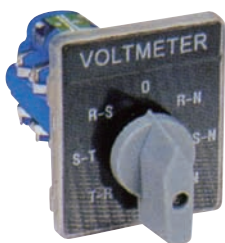
CS-68-20A (volt meter)
